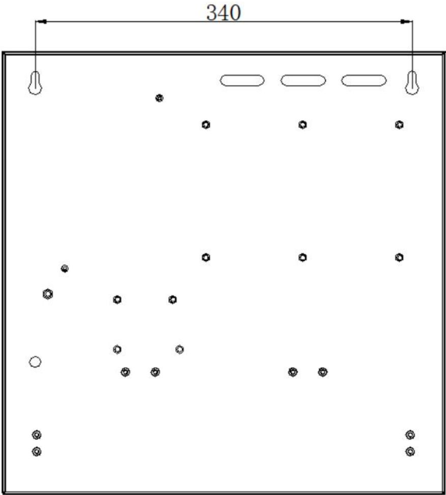
图 2-7 壁挂安装尺寸
