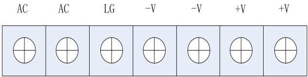
图 2-6 电源端子
