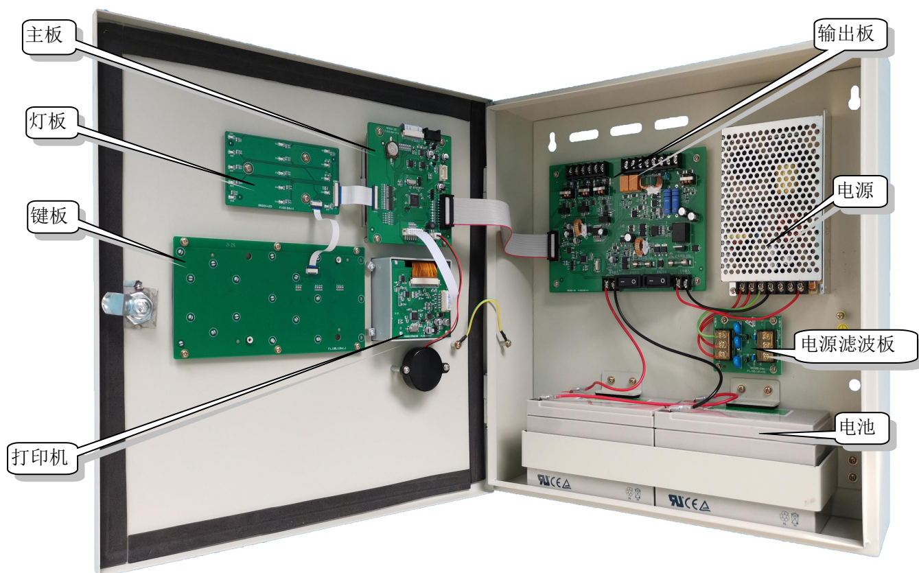
图 2-2 内部结构与连接
