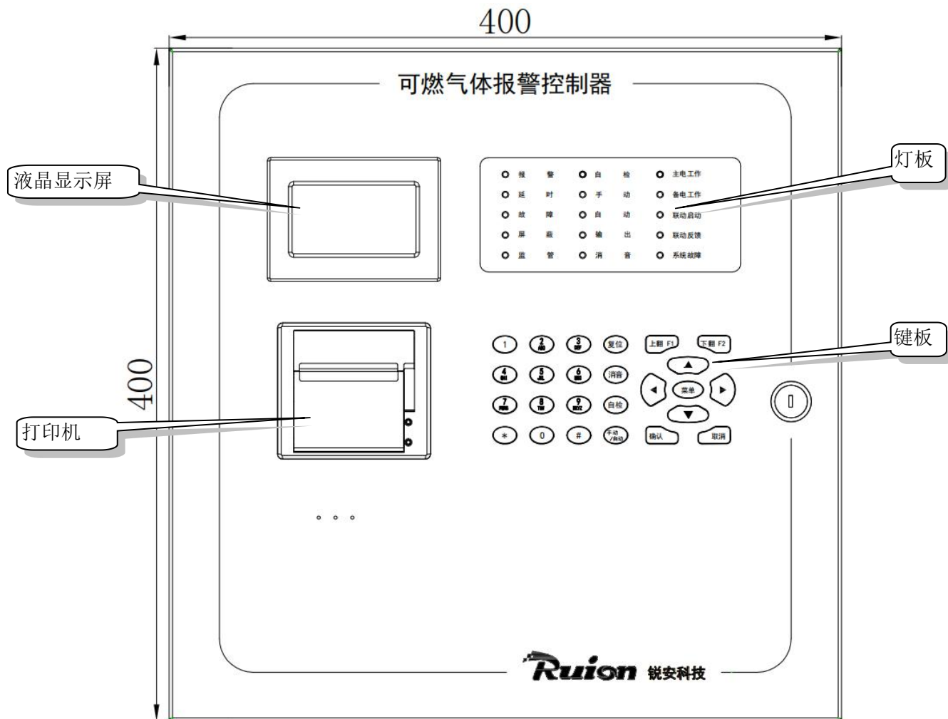
图 2-1 外观示意图
