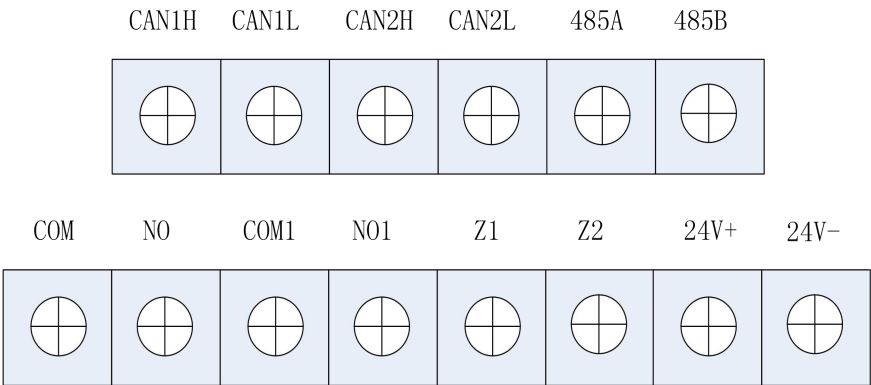
图 2-4 输出板对外端子
