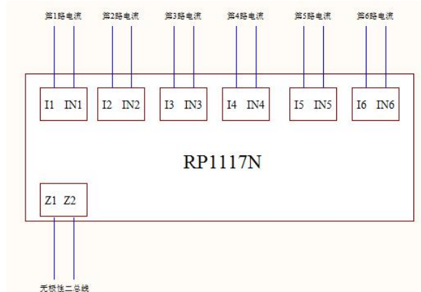
图 3 传感器接线示意图
