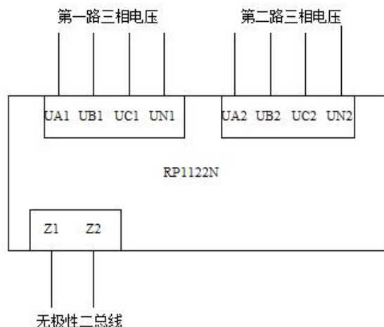
图 2 传感器接线示意图
