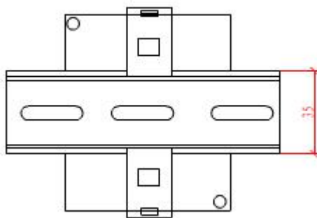
图 2 传感器安装方式
