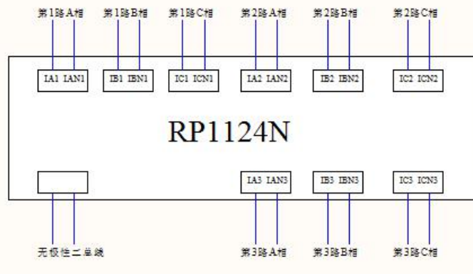
图 3 传感器接线示意图
