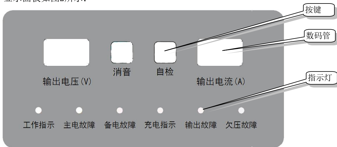
图2 按键及显示面板示意图
