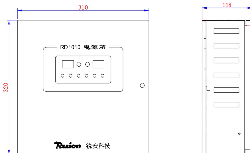
图1 外形示意图
