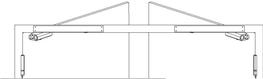
推门面安装位置标示（单位 MM）
