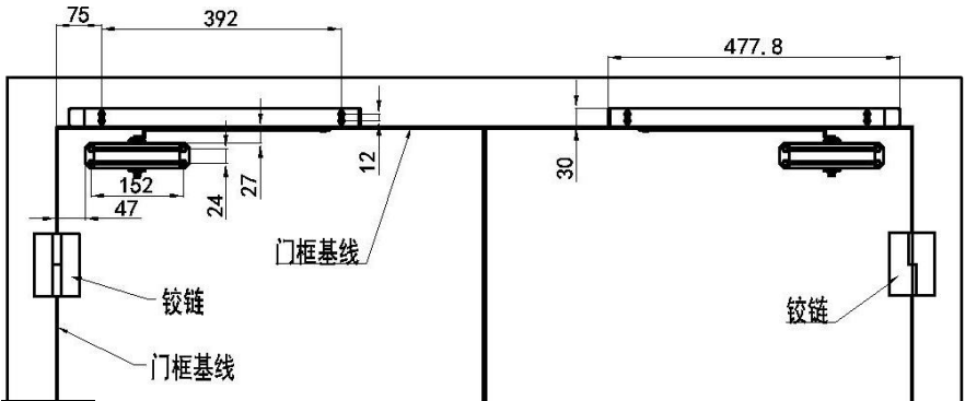
推门面安装位置标示（单位 MM）
