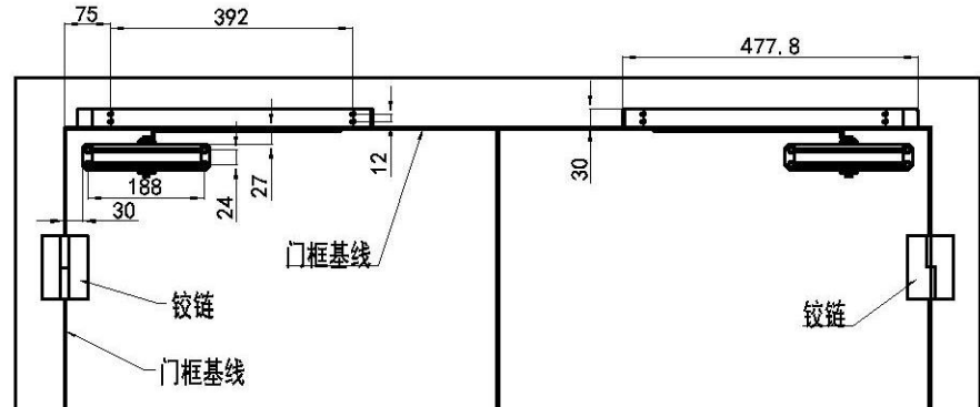
推门面左开门安装步骤（人在门里往外推门）
