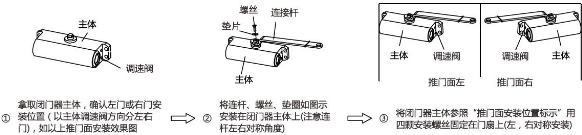
推门面左开门安装步骤（人在门里往外推门）
